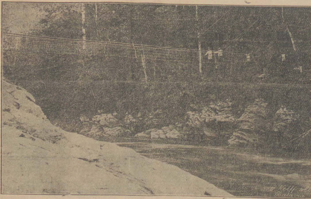
ROTTANBRUG OVER DE KORORIVIER (MIDDEN-CELEBES)
